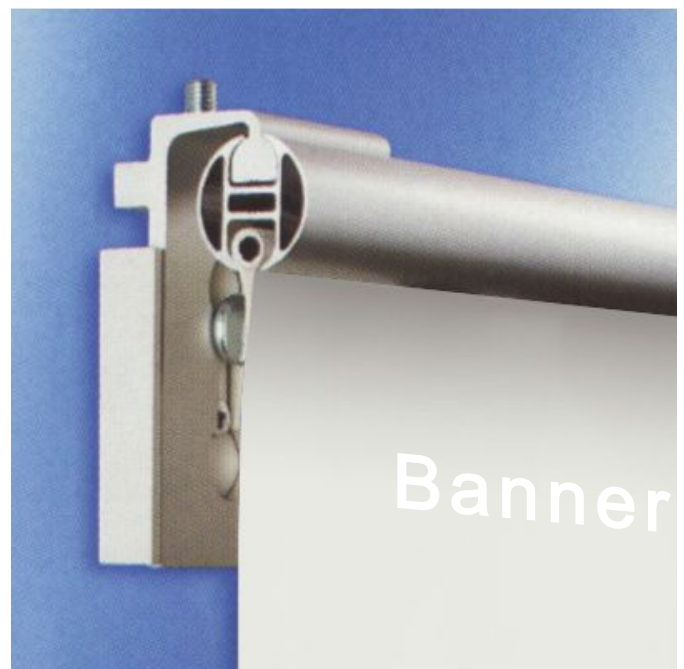
Wandhalterung für Aluminium-Schiene rund D. 30 mm
